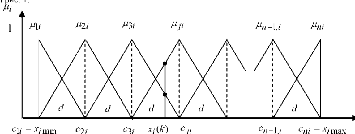
Рис. 1. Трикутні функції належності нео-фаззі нейрона
