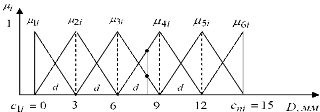
Рис. 3. Функції належності вхідної змінної «Дефіцит вологості повітря»
